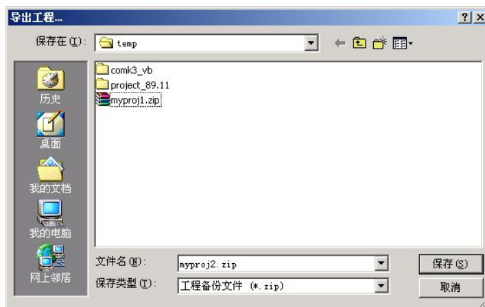
图 2-4 导出工程
