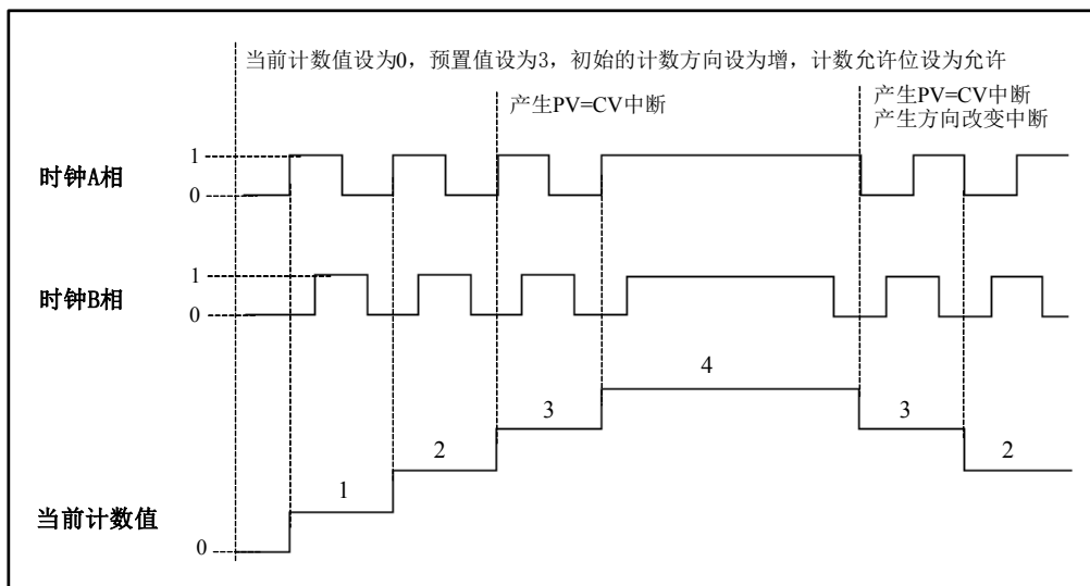
图 6-7 模式 9、10、11 的时序图（正交，1x）
