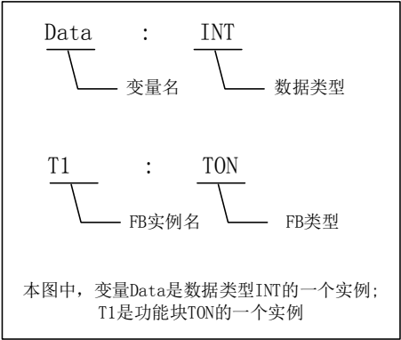
图 3-1 实例化举例
