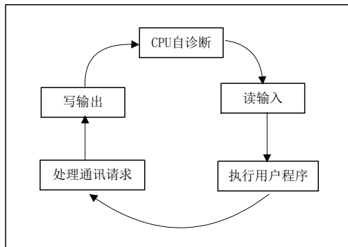
图 2-7 扫描周期
