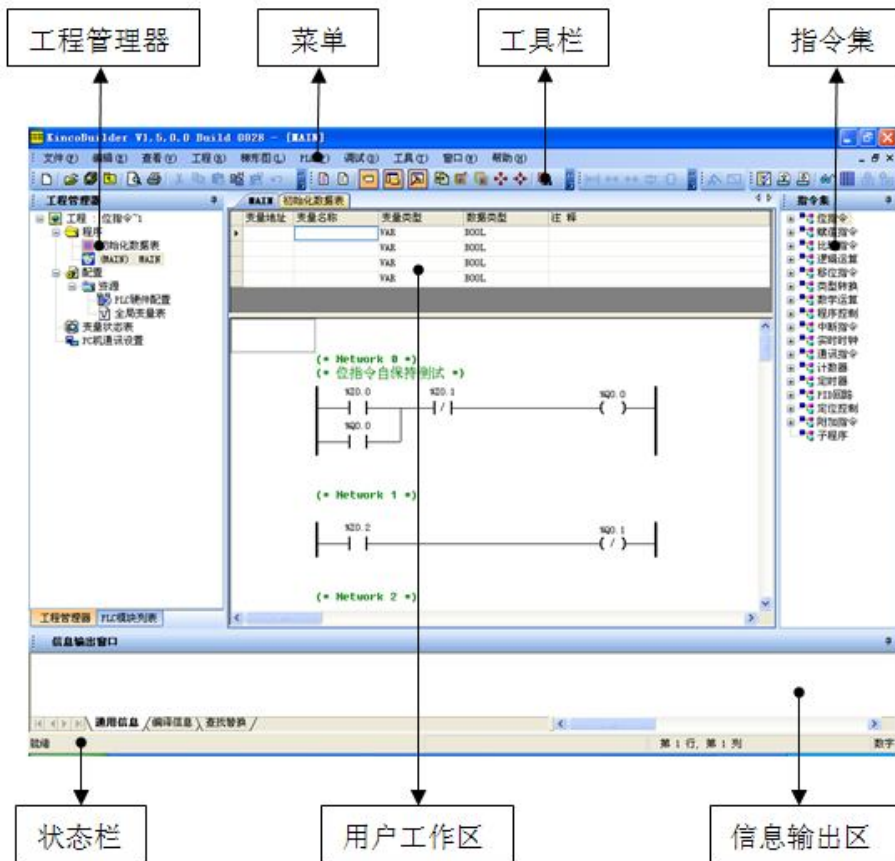
图 2-3 KincoBuilder 界面
