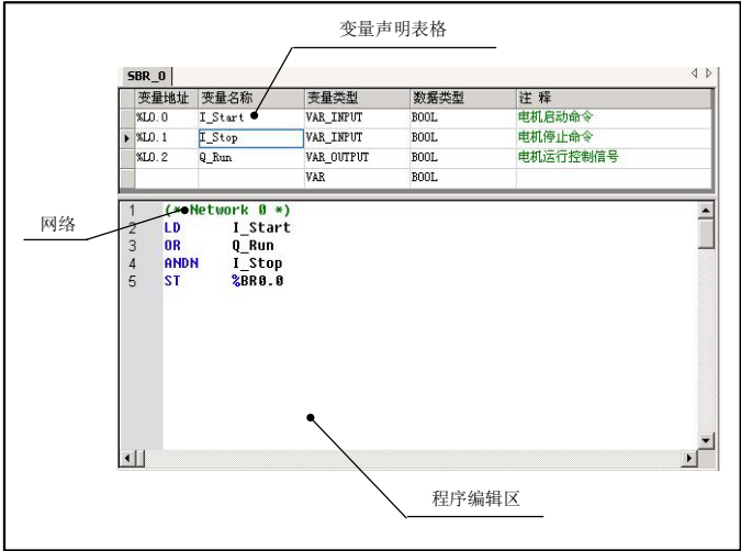
图 5-1 IL 编辑器
